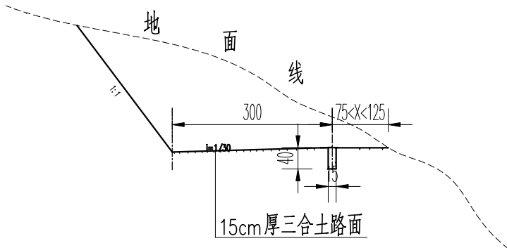
0+032-0+120 I 型路面 1: 100
