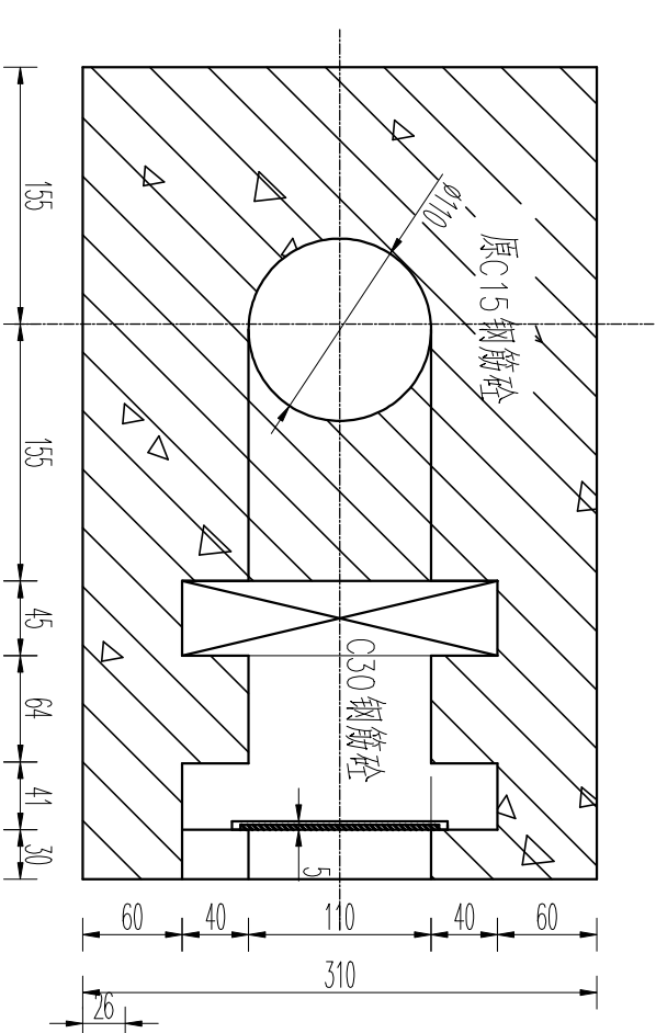
C-C剖面
