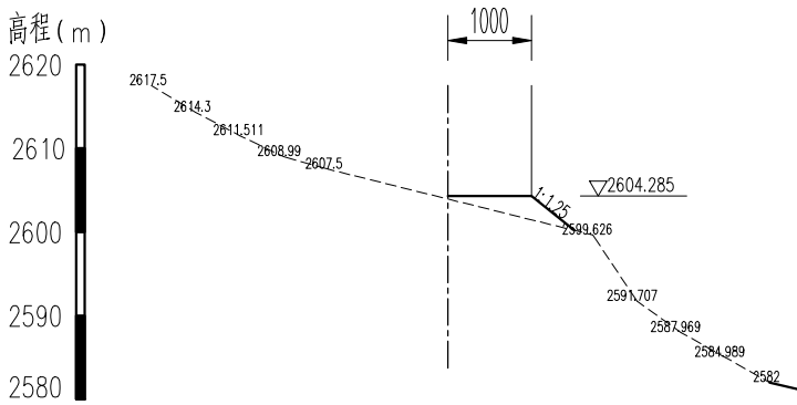
KA13-0+119.63 1: 1000
