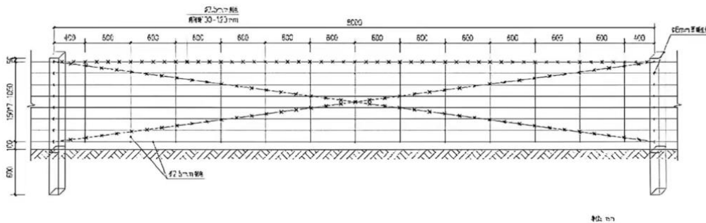
“7+1” 水泥桩刺丝围栏示意图
